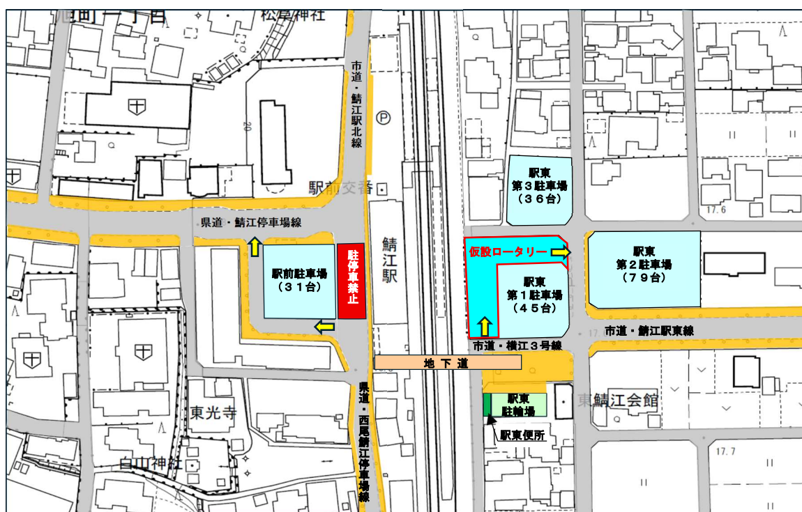
図2：実験中の駅周辺配置図
