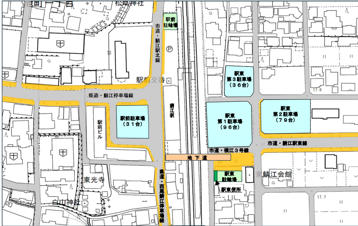
図 1：現況の鯖江駅周辺配置図
