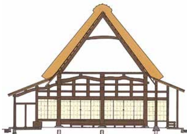
梁間断面図 S≒1/210
