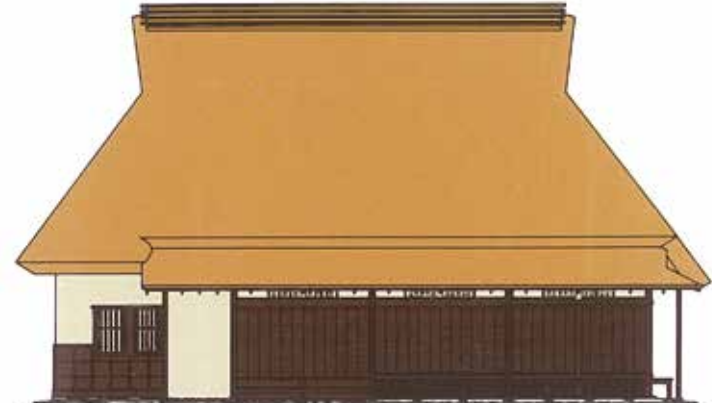
南側立面図 S≒1/210
