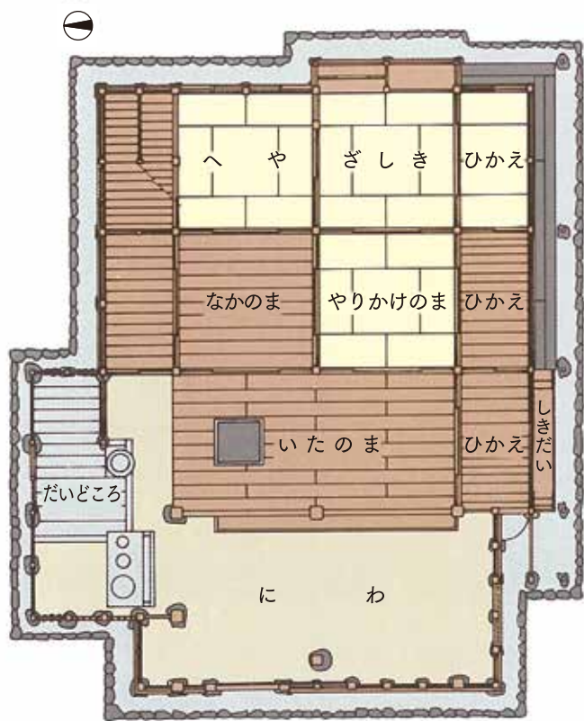
平面図 S≒1/150
