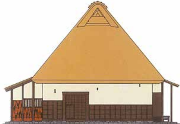
正立面図 S≒1/210
