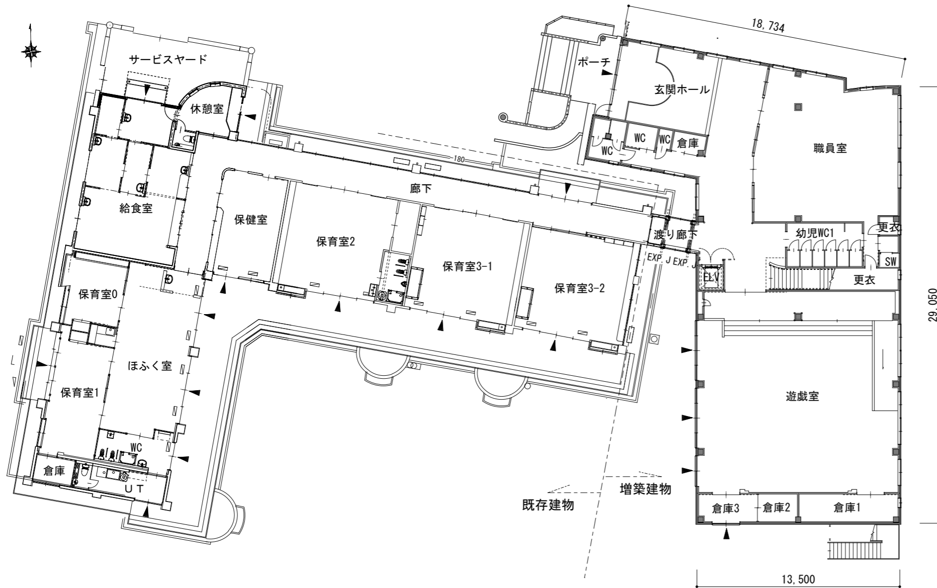
1階平面図
