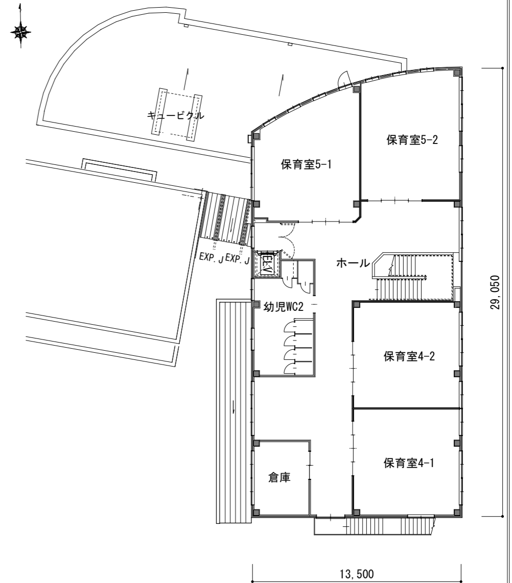
2階平面図
